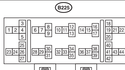
继电器支架
